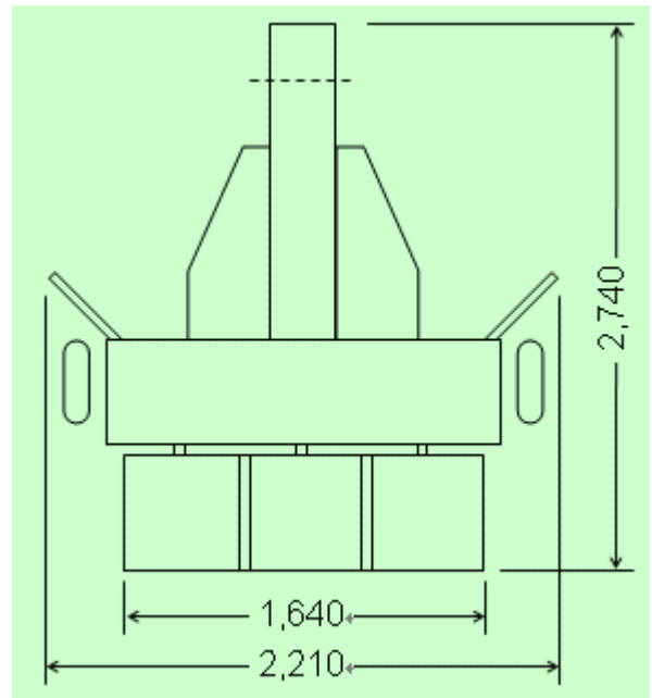
集球ドラム3連仕様
