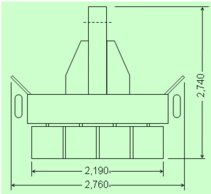
集球ドラム4連仕様
